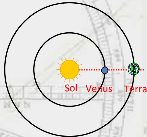
En un trànsit, Venus, el Sol i la Terra estan alineats
